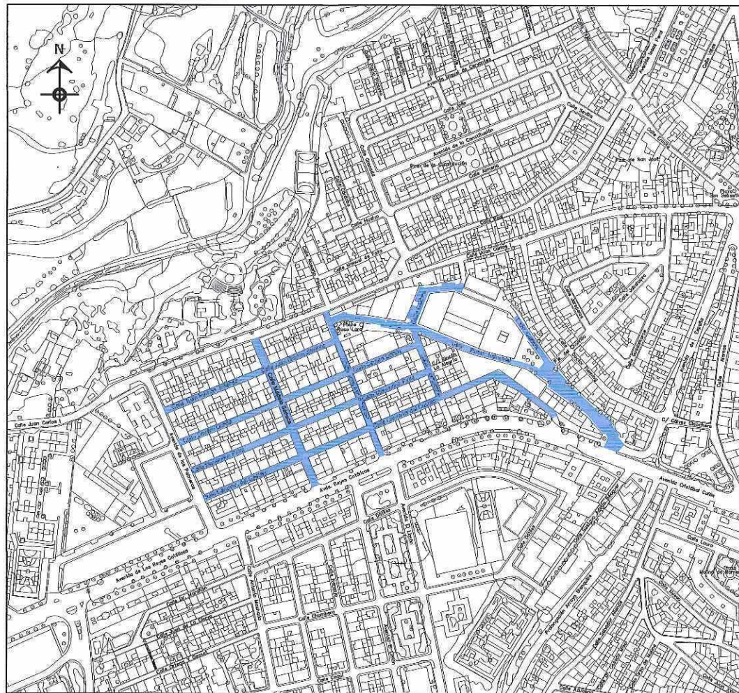
PLANTA DE LAS OBRAS EN BARRIO LA ALEGRÍA Y ZONA AYUNTAMIENTO
