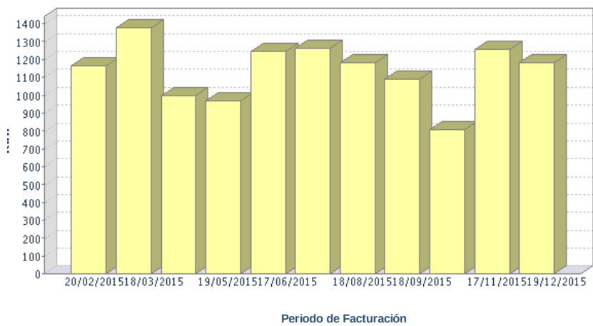
Consumo de energía reactiva (kVarh)
